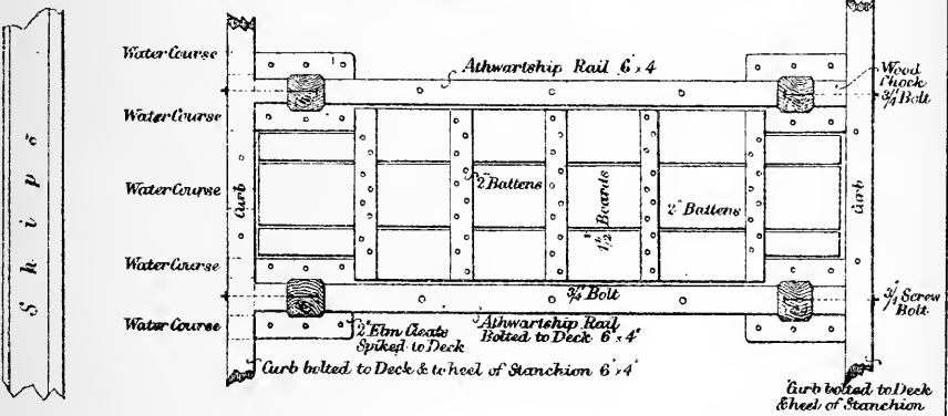
PLAN A.A
